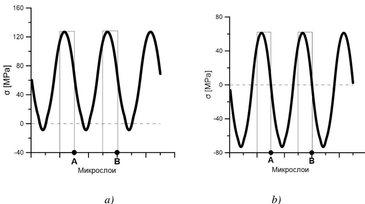
Рисунок 14 – Распределение остаточных напряжений.
