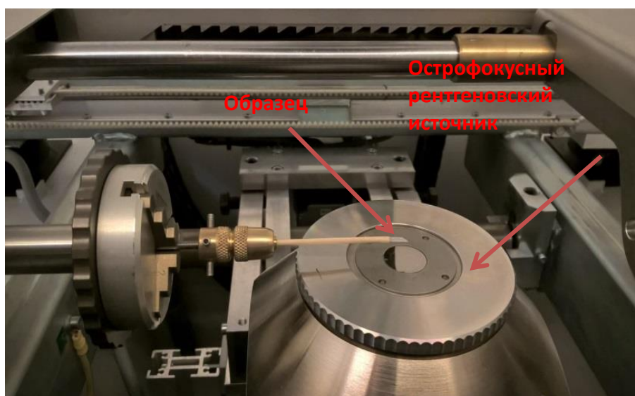
Рисунок 27 – Образец спеченного слоя низкотемпературной керамики в испытательной камере.
