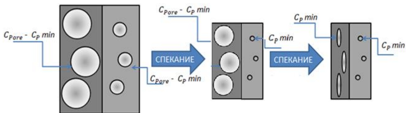
Рисунок 6 – Схема механизма усадки спеченного тела ( C_{pore} - C_p min > 0 – условие сферически-симметричного сжатия материала).
